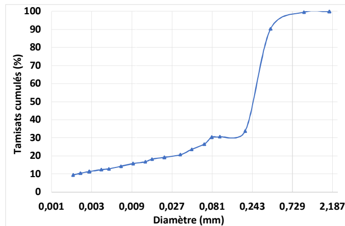
Figure 1: Courbe granulométrique des sédiments marins
