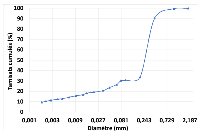
Figure 1: Courbe granulométrique des sédiments marins
