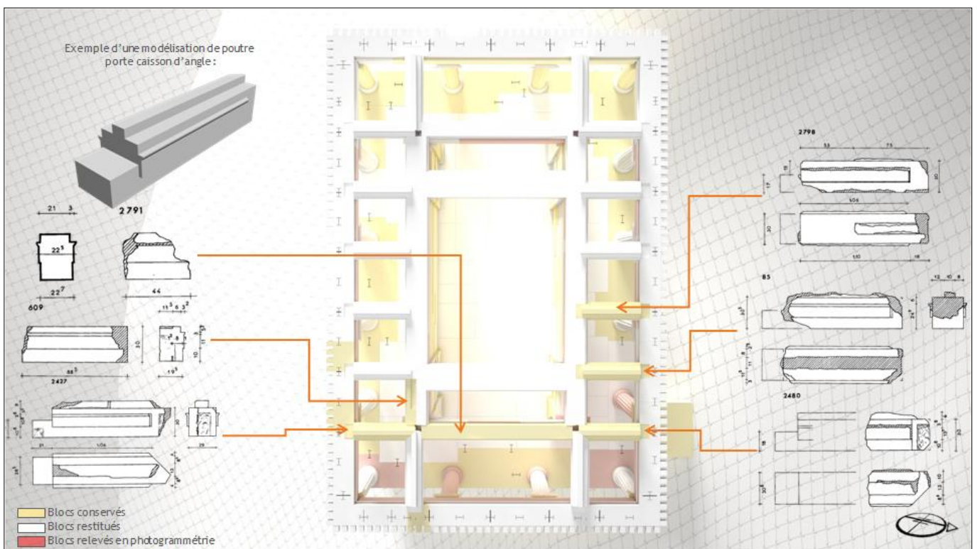
Figure 25 : Disposition retenue pour la restitution des poutres portes caissons, ainsi que les longirons.
