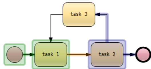
Fig. 2. Infinite loop.
