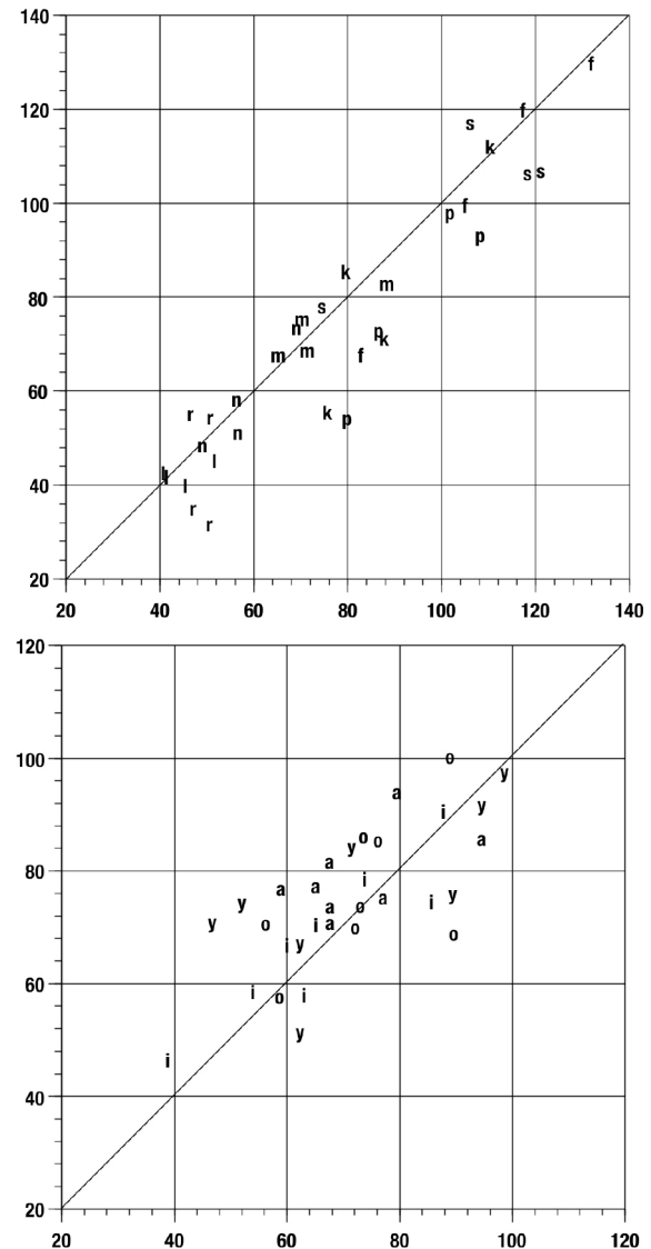
Figure 1: Diagrammes de dispersion pour les durées de C_p (haut) et V_2 (bas). En abscisse, les durées pour CCV#CVCV, en ordonnée, pour CCVC#VCV. Les données correspondent à la moyenne des deux répétitions pour la première mention.
