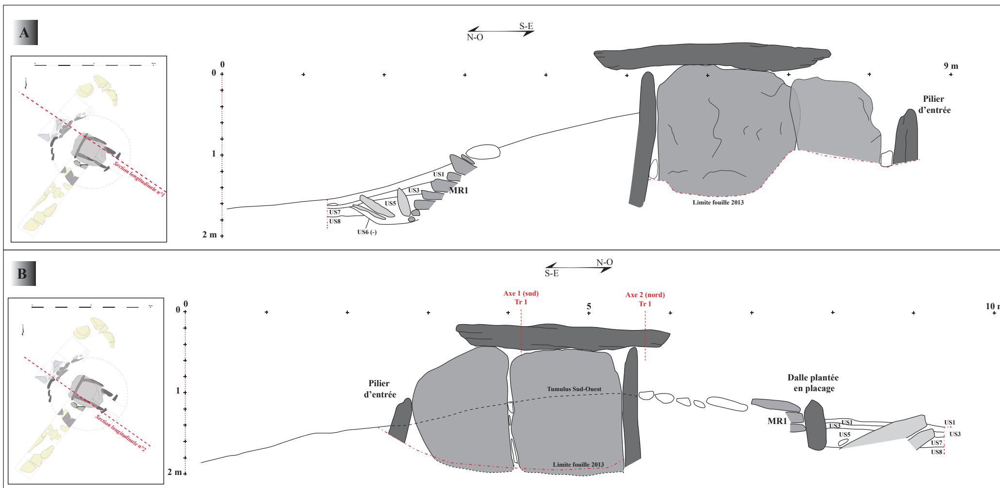
Figure 72 : Sections longitudinales passant par les parois latérales de la chambre et le sondage 3.
