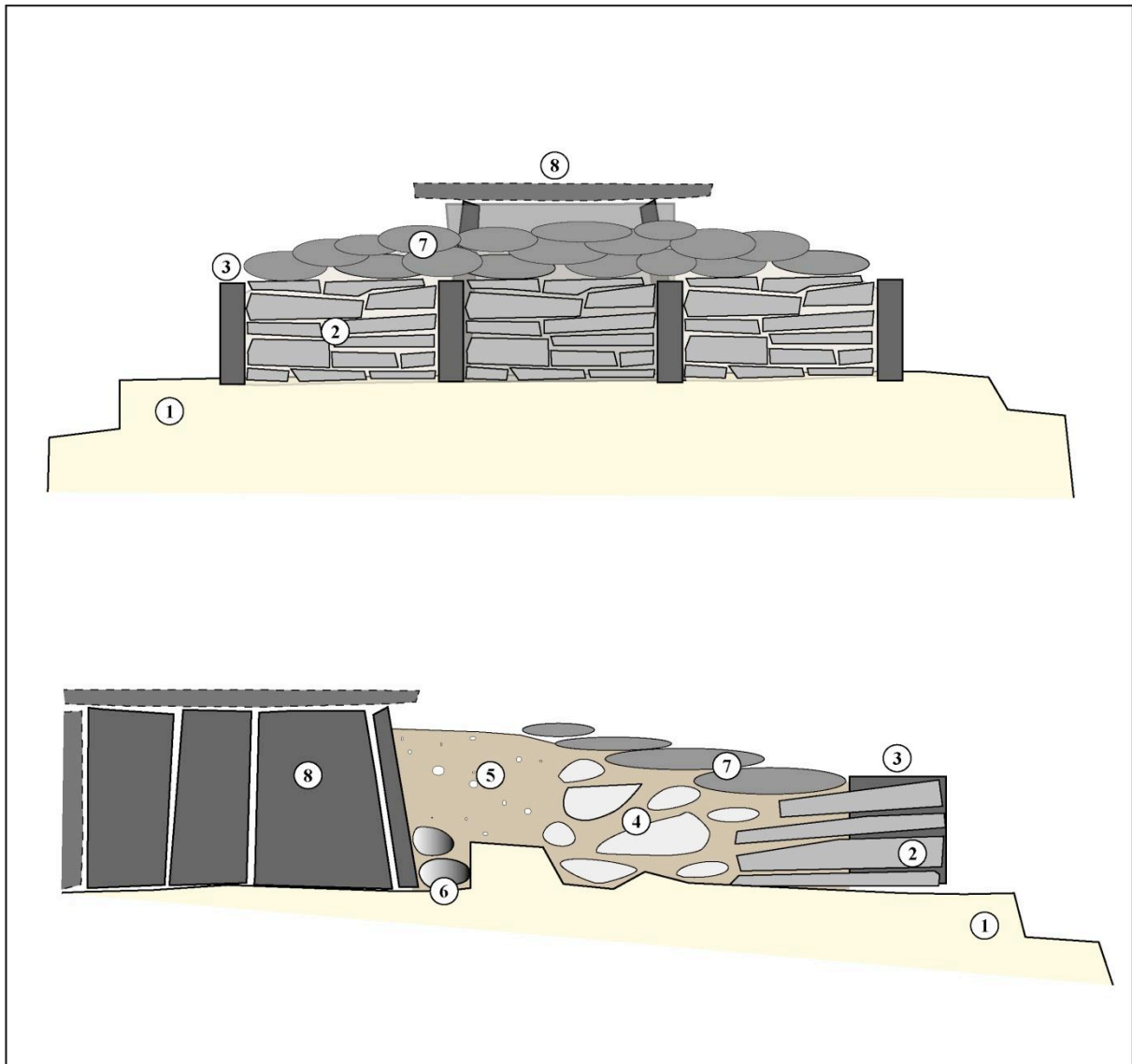
Figure 105 : Dolmen de Prat-Clos, hypothèse de restitution de la structure tumulaire. 1 : Substrat ; 2 : MR1 ; 3 : Dalle plantées rayonnantes ; 4 : Remplissage de blocs et de terre (US5) ; 5 : Remplissage de terre (US6) ; 6 : Calage de l'orthostate ; 7 : Dalle en écaille (US4) ; 8 : Chambre sépulcrale.
