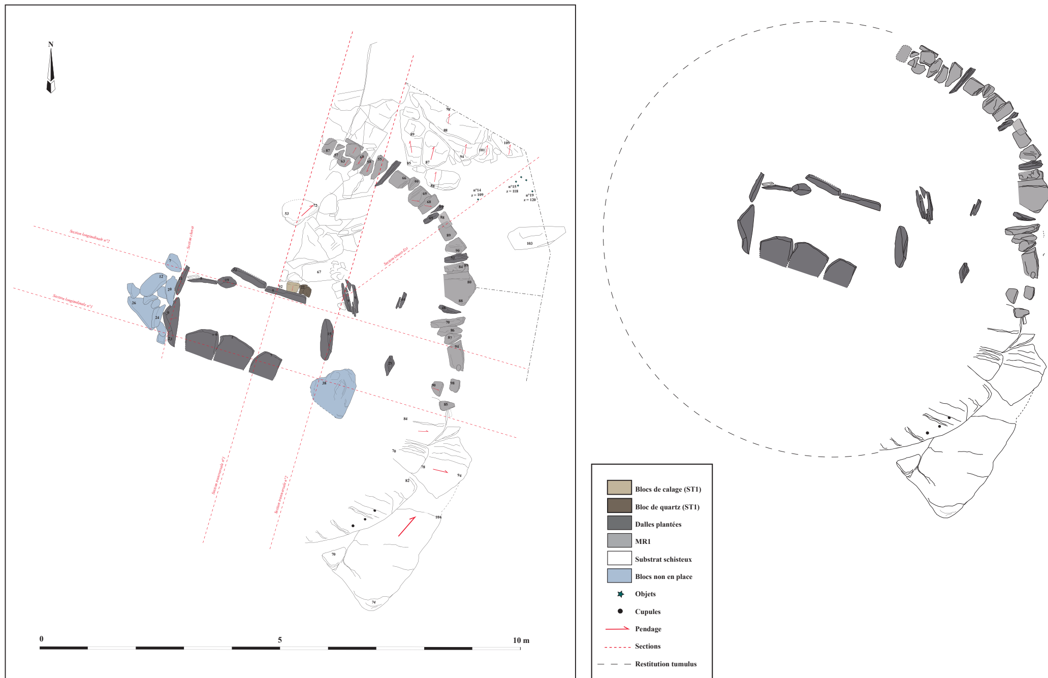
Figure 22 : Planimétrie générale du Dolmen de Prat-Clos. A droite : reconstitution hypothétique du parement du tumulus.
