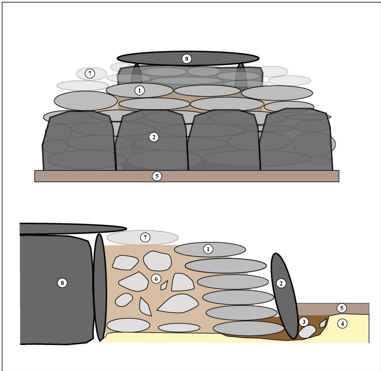
Figure 106 : Dolmen de la Barraca, hypothèse de restitution de la structure tumulaire. 1 : MR1 ; 2 ; Dalle plantée en placage contre MR1 (péristalithe) ; 3 : Tranchée de fondation pour l'implantation de 1 et 2 ; 4 : Arène granitique, niveau de fondation du monument ; 5 : Sol postérieur à la construction ; 6 : Remplissage interne derrière MR1 ; 7 : Hypothèse de hauteur originel du tumulus ; 8 : Chambre sépulcrale.
