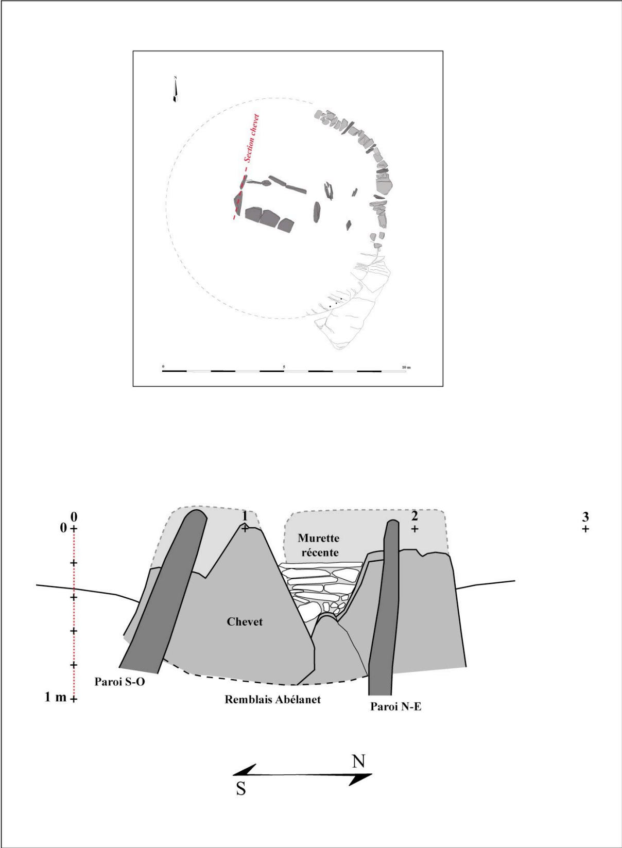
Figure 20 : Section transversale Nord-Sud de la chambre sépulcrale par le chevet.
