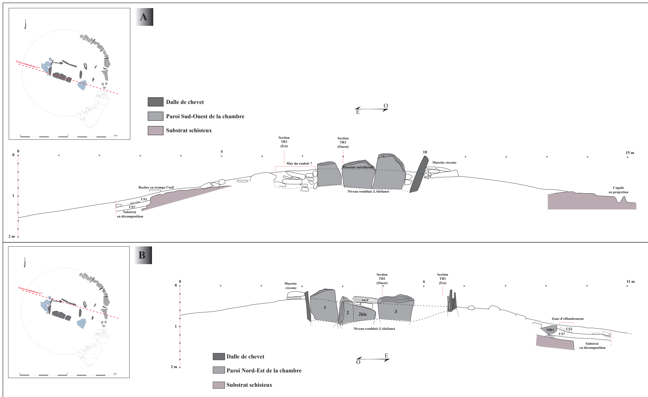
Figure 17 : Sections longitudinales du dolmen de Prat-Clos. A : Section Est-Ouest passant par la paroi sud-ouest de la chambre. B : Section Ouest-Est passant par la paroi Nord-Est de la chambre
