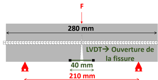
Figure 2. Flexion trois points sur une éprouvette de 70 \times 70 \times 280 mm
