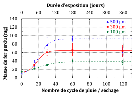
Figure 8. Evolution de la masse de fer perdu en fonction du nombre de cycle de pluie / séchage et des ouvertures de fissure résiduelle
