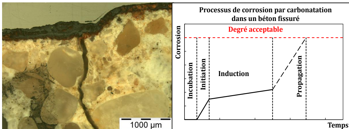
Figure 11. Photo au microscope optique d'une fissure dans un échantillon ayant une fissure résiduelle de 100μm après 60 cycles de pluie / séchage
