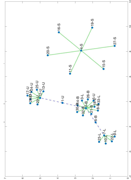
Figure 7 – Clustering du jeu de données Cars en 4 classes ( \epsilon = 0, 25 ).
