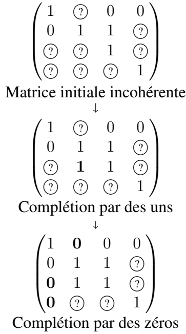
Figure 4 – Déduire des éléments de la matrice.
