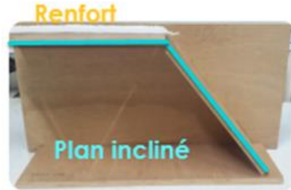
Fig. 3. Dispositif « KES ».
