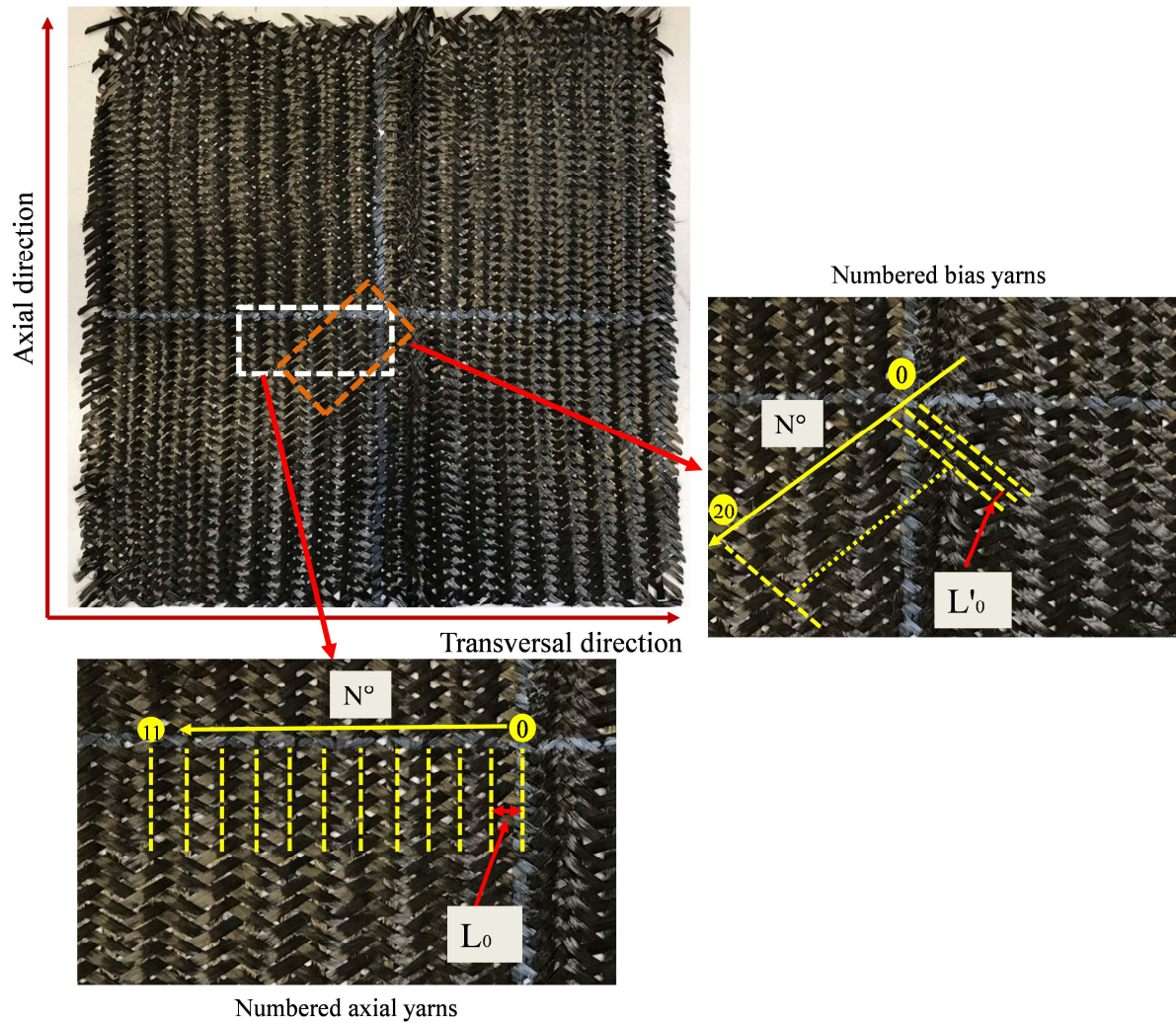
Fig. 4. Renfort tressé avant le préformage.
