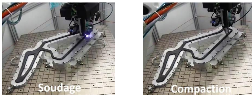
Figure 8 : Exemple d'application du procédé AREVO dans la confection d'un cadre de vélo en composite fibre de carbone, avec à gauche l'étape de soudage laser des différentes couches et à droite l'étape de compaction[17].
