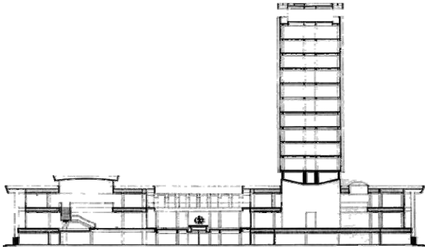
Figure 5.2. Ouvrage – coupe verticale
