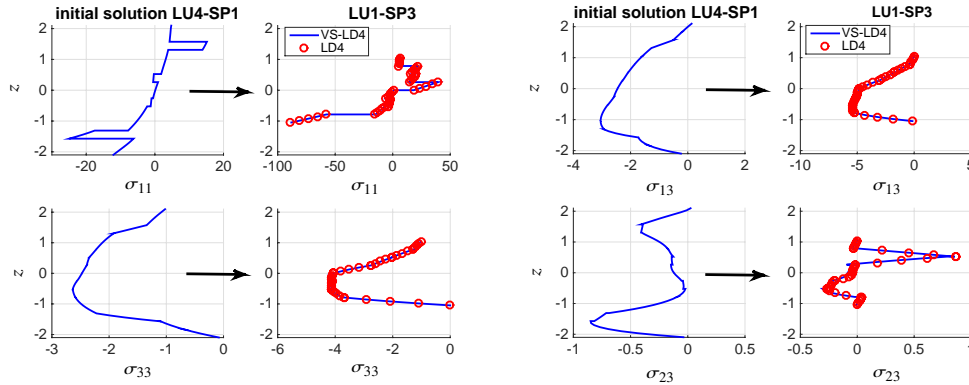
Fig. 5. Distribution de \sigma_{11} , \sigma_{13} , \sigma_{33} dans l'épaisseur - Processus multi-résolution à partir des fonctions de base associées à LU4-SP1 [ 45_2^0/0/-45_3^0/90/45 ] s - nouveau stratifié LU1-SP3 : [ 0^0/45^0/90^0/-45^0/0/45^0/-45^0/90^0 ]
