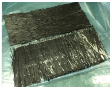
Fig. 7.a bandes de FCrR assemblées pour réaliser un pseudo NCF 0°-90°
