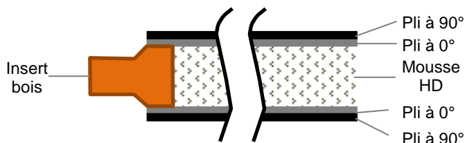
Fig. 7.b Schéma de drapage de la porte de roof
