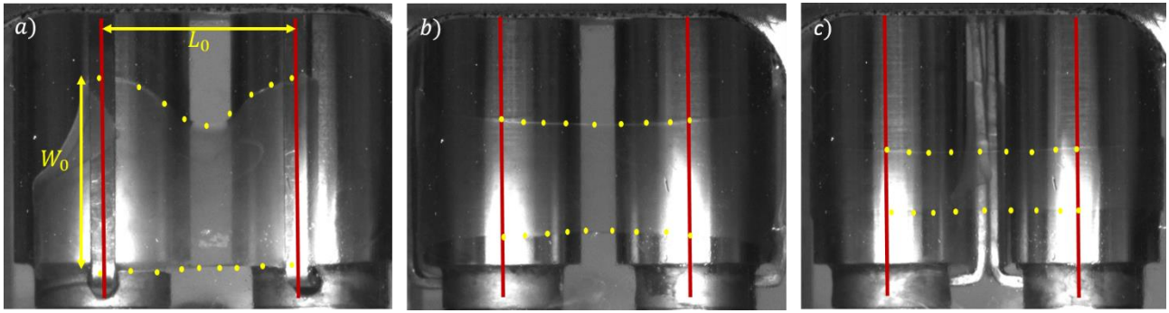
Fig. 5. Mesure d'extension à 200^{\circ}\text{C} , pour un taux de déformation Hencky de 0,5 \text{ s}^{-1} , les lignes rouges représentent la distance L_0 a) t=0 \text{ s} , l'échantillon n'est pas étiré, b) t=3 \text{ s} , l'échantillon est en cours d'extension, c) t=7,726 \text{ s} , fin de la mesure au moment du contact des agrafes
