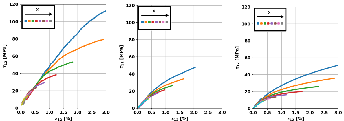
Fig. 8. Identification du comportement d'interface en considérant un comportement élastique des bras pour un matériau composite [0]_{16} à a. température ambiante, b. 70^\circ\text{C} et c. 100^\circ\text{C} .
