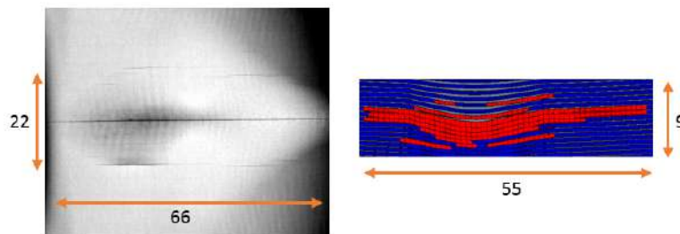
Fig. 10. Endommagement du pli 1 (pli opposé à l'impact)
