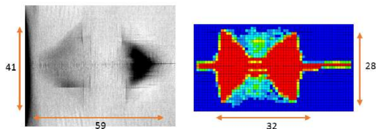
Fig. 11. Délaminage entre les pli 1 et 2
