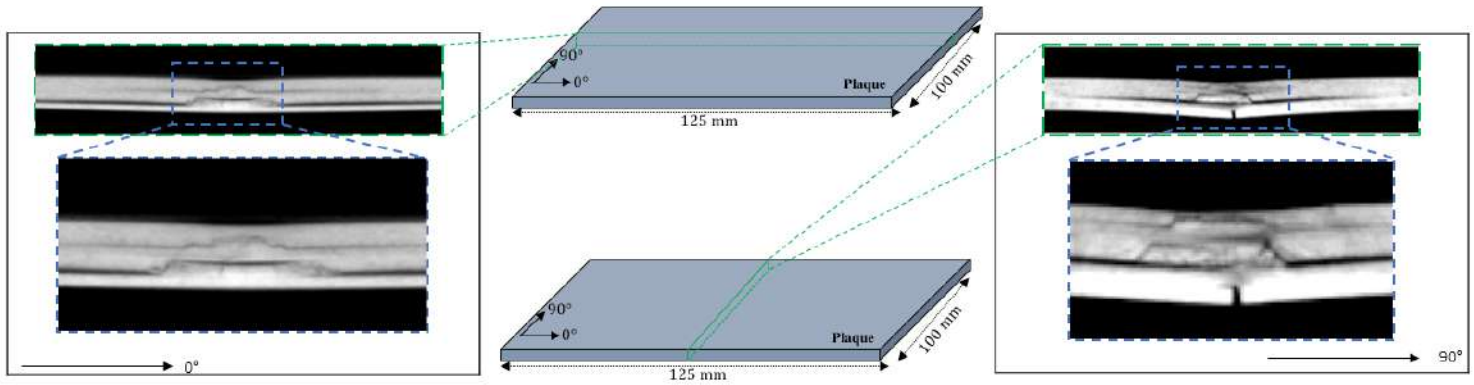
Fig. 5. Endommagements sur les plis supérieurs (Configuration C1)
