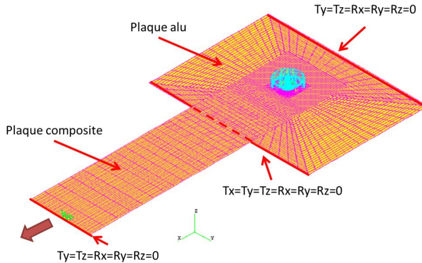
Fig. 3. Maillage et conditions aux limites pour la simulation d'un essai de simple cisaillement soutenu
