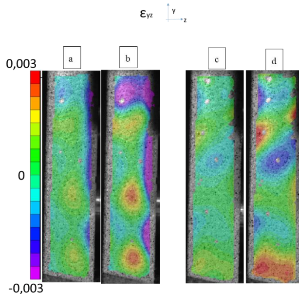
Fig. 3. Déformation de cisaillement pour les composites : R7 à des niveaux de contraintes respectives (a)200MPa (b) 350MPa, et R8 à des niveaux de contraintes respectives (c) 200MPa et (d) 350MPa.
