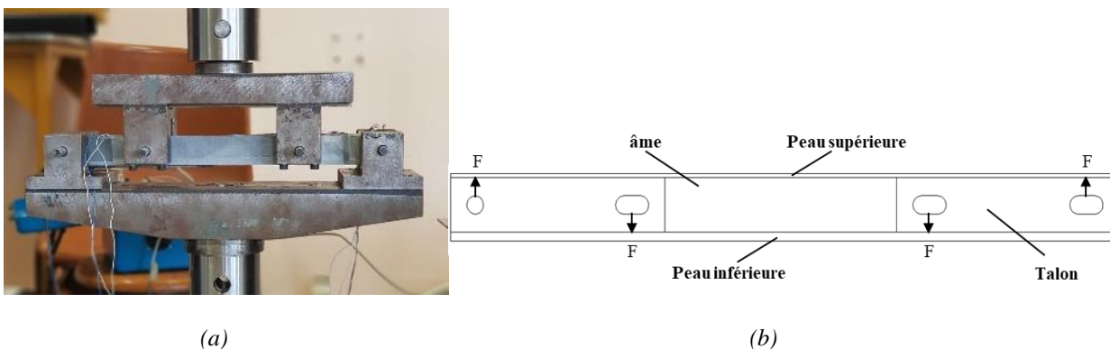
Fig. 1. (a) le montage de l'essai flexion 4 points (b) Géométrie de l'éprouvette.
