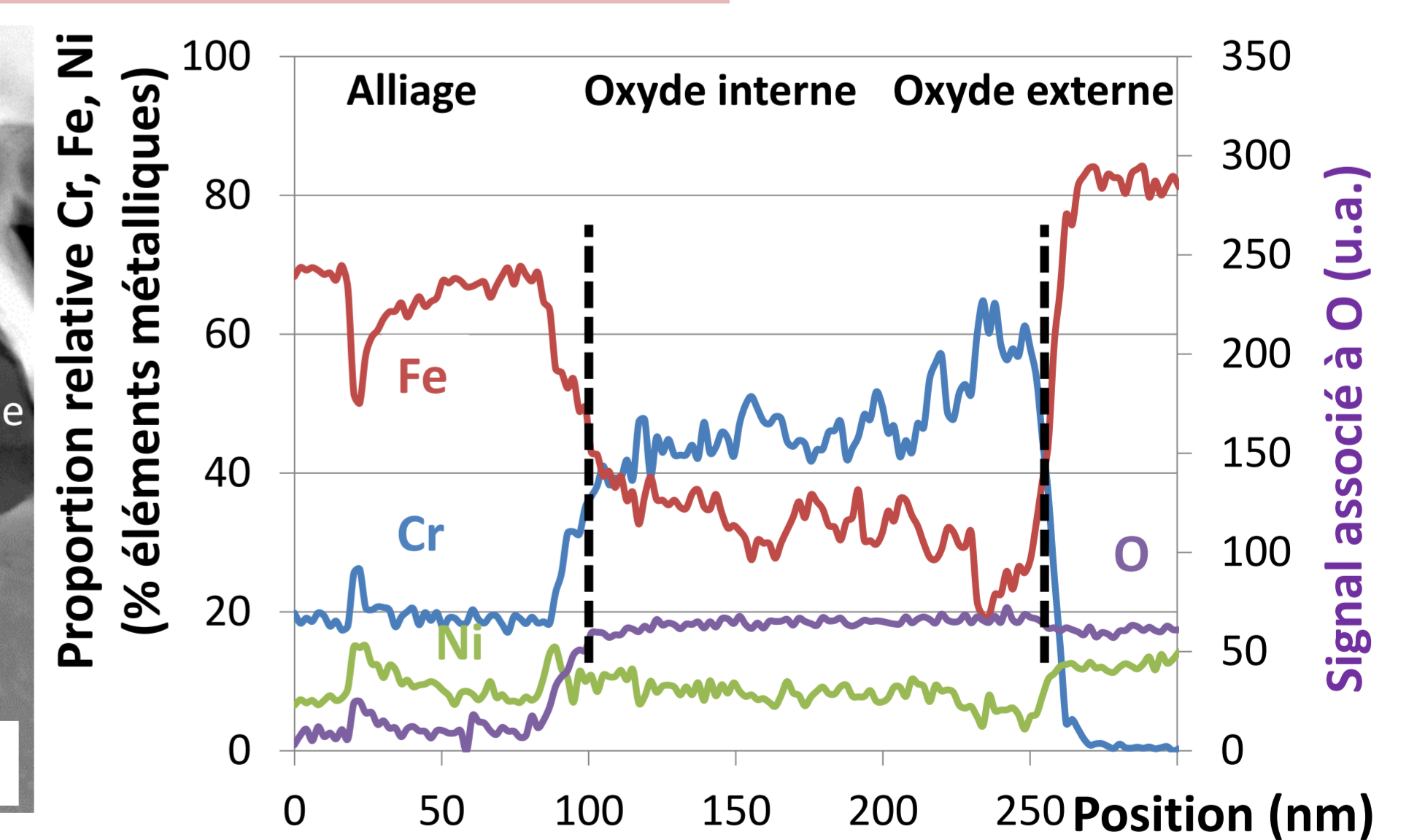
Cliché STEM-HAADF des couches d'oxyde de surface et profils EDX correspondants, échantillon C2
