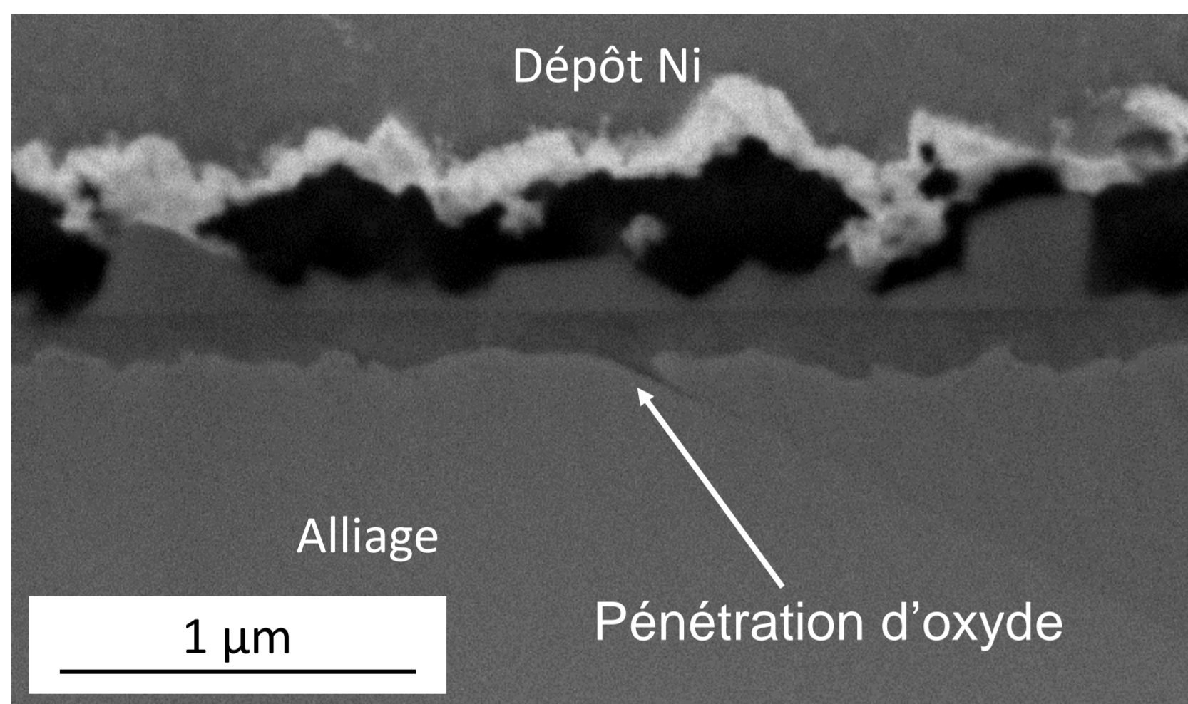
Cliché MEB en coupe transverse (électrons rétrodiffusés), coupon C2
