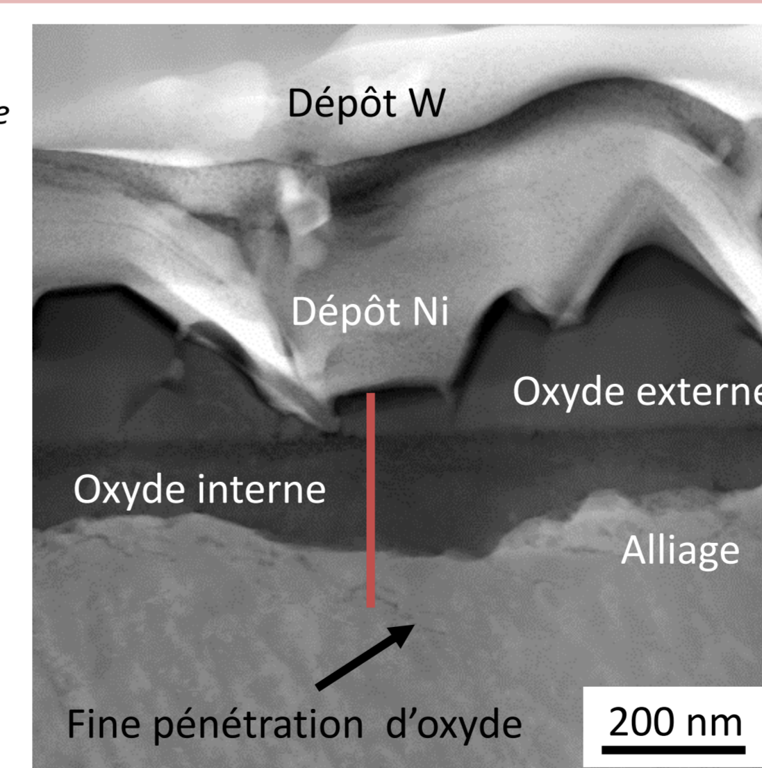
Cliché STEM-HAADF des couches d'oxyde de surface et profils EDX correspondants, échantillon C2
