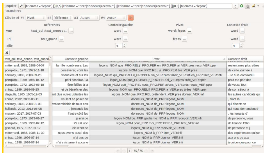
Figure 2 - Concordance sur les occurrences du prédicat tirer/donner/recevoir avec l'argument leçon(s) , triée par construction de surface (séquence de catégories grammaticales) puis par date.
