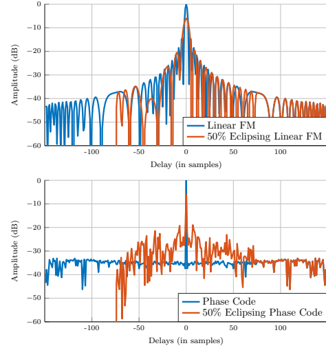
FIGURE 2 – Séquence de corrélation pour un signal éclipse En haut : un chirp. En bas : un code de phase. Notez l'épaississement du lobe principal pour le chirp, la remontée des lobes secondaires pour le code de phase, et la perte due à la désadaptation.
