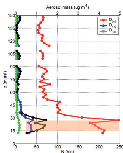
Figure 2. Profils verticaux des concentrations moyennes en masse (courbe noire, axe du haut) et en nombre de particules de tailles supérieures à 0,5, 1,0 et 3,0 \mu\text{m} de diamètre (respectivement courbes rouge, bleue et verte, axe du bas, en particules par \text{cm}^3 ) des aérosols au-dessus de la zone de déferlement. La zone orange représente la gamme des mesures instantanées de la masse d'aérosols dans la couche de surface ( z < 30 m d'altitude).
