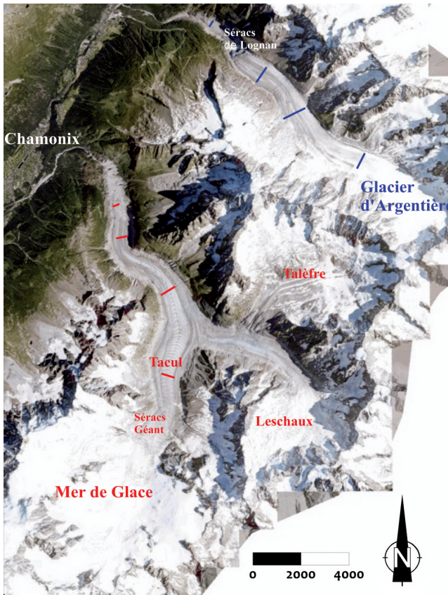
Figure 3. Carte des glaciers d'Argentière et de la Mer de Glace. Les lignes représentent les sections transversales mesurées depuis la fin du XIX e siècle (figure 5) (profils 7, 5, 4 et 2 du haut en bas pour le glacier d'Argentière et profils Tacul, Trélaporte, Echelets et Montenvers pour la Mer de Glace). L'arrière-plan est une orthophoto-aérienne de l'Institut national géographique datant de 2015 ( https://www.geoportail.gouv.fr/ ).
