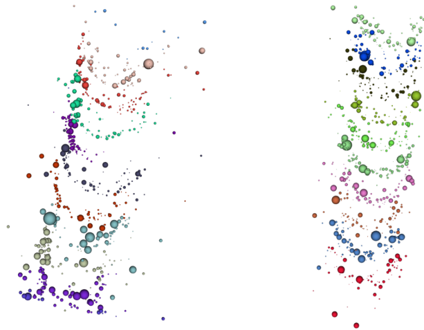
FIGURE 4 – Population de défauts observée (à gauche, les défauts sont représentés par leur sphère équivalente) et simulée (à droite).
