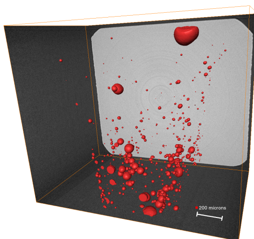
FIGURE 2 – Reconstruction 3D des images de tomographies obtenues au Synchrotron SOLEIL. Tous les volumes rouges représentent des défauts. Le voxel est un cube de 1,3\mu\text{m} de coté.
