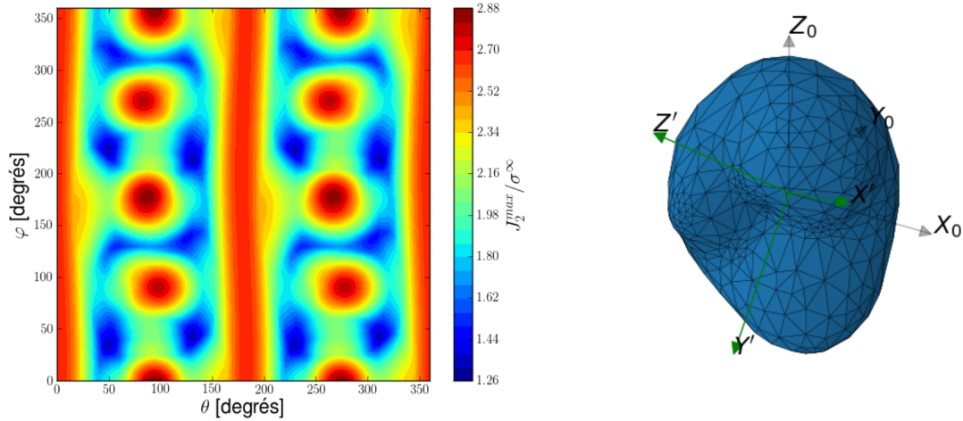
FIGURE 3 – Carte de concentration de contrainte équivalente de von Mises du défaut représenté à droite sollicité en traction simple dans la direction \underline{d} = (\cos(\varphi) \sin(\theta), \sin(\varphi) \sin(\theta), \cos(\theta))^T .
