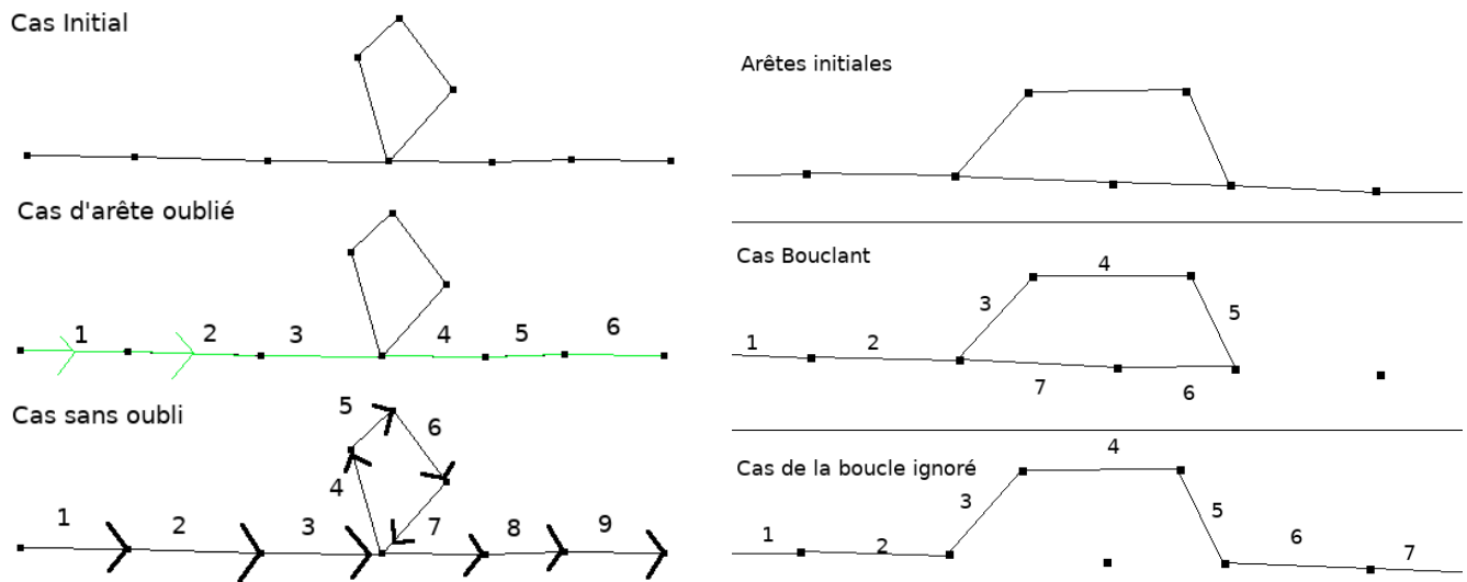
FIGURE 20 – Scénario possibles liés à la présence d’une boucle dans la bordure.
