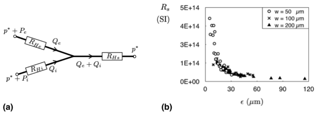
FIGURE 3 – (a) Représentation du circuit par analogie électrique. (b) Résistance R_s de la branche de sortie en fonction de la largeur \epsilon du jet.
