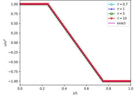
(d) horizontal velocity obtained with the VP MRT LBM
