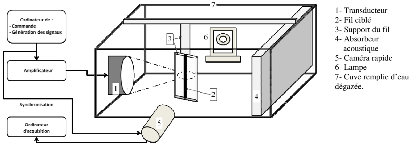
FIG. 1 – Schémas du principe du dispositif expérimental.
