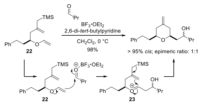
Scheme 13. Aldol– Prins cyclisation cascade.
