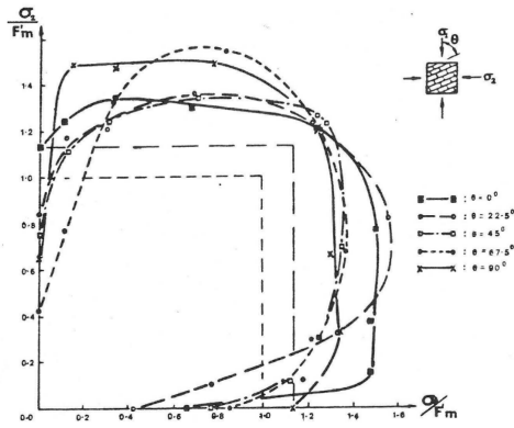
(a) Surface de rupture en contraintes biaxiales [11]
