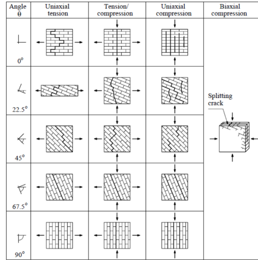
(b) Faciès de fissurations sous sollicitations biaxiales [7]
