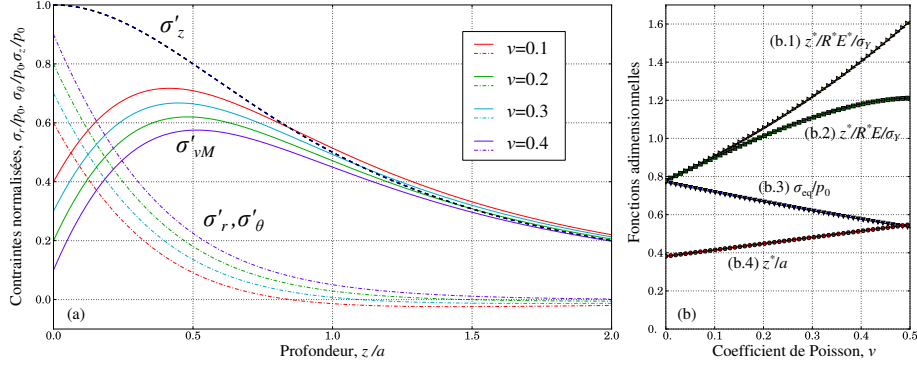
Figure 1.7. (a) Contrainte \sigma_\theta , \sigma_r et \sigma_z le long de l'axe de symétrie ; (b) des fonctions adimensionnelles qui représentent (b.1) la profondeur normalisée de commencement d'écoulement plastique z^*/R^*E^*/\sigma_Y , (b.2) la profondeur normalisée dans le cas d'indenteur rigide z^*/R^*E^*/\sigma_Y , (b.3) la contrainte de von Mises maximale normalisée \sigma_{eq}/p_0 , (b.4) la profondeur normalisée z^*/a , la solution d'Eq. [1.16] ; les lignes solides dans (b) représentent des solutions approximatives [1.19],[1.20],[1.18],[1.17], respectivement.
