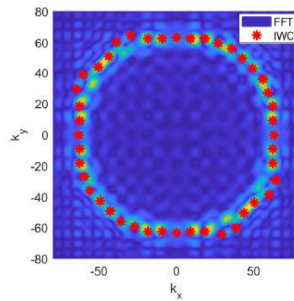
(d) Comparison FFT-IWC at 1100.0 Hz.
