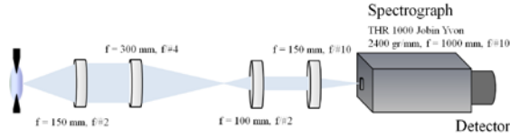
Fig. 2 : Dispositif de spectroscopie d'émission
