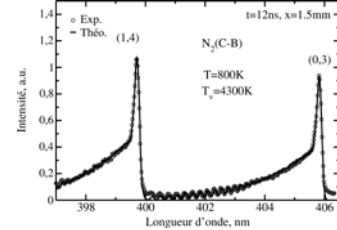
Fig. 4 : Comparaison entre un spectre expérimental et un théorique de \text{N}_2 (C-B)
