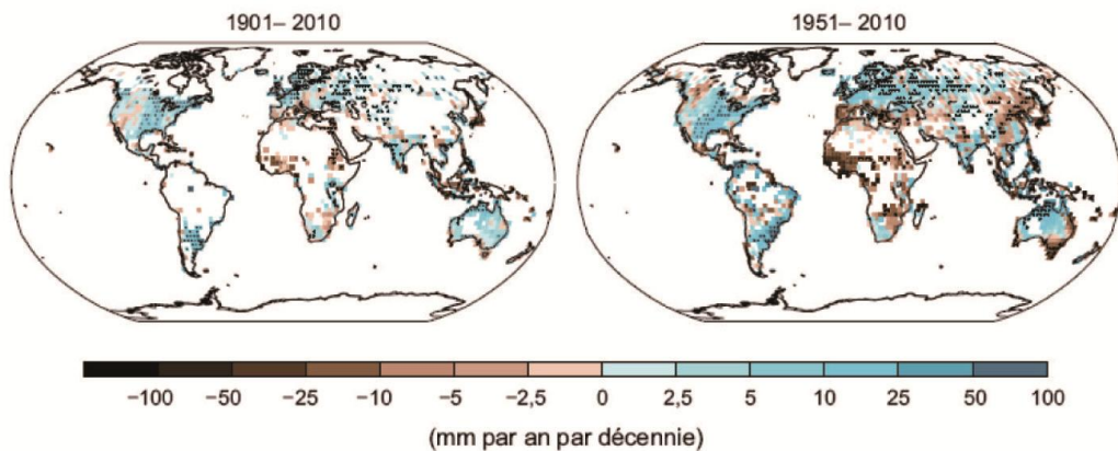
Figure 3: Changements observés des précipitations annuelles sur les terres émergées. Source: IPCC, 2013
