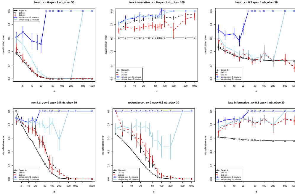
Figure 1: Influence du nombre de variables sur l’erreur de classification pour les différents scénarii. Première ligne C1 (gauche), C2 (centre), C3 (droite); deuxième ligne C4 (gauche), C5 (centre), C6 (droite). Sont représentées l’erreur de Bayes (trait plein noir), l’erreur empirique avec la méthode MixDiag (trait plein cyan), avec MixCor (trait plein bleu sombre), avec cc21 (pointillé noir), avec cc22 (pointillé rouge). Moyenne faite sur 30 échantillons de 2 \times 15 observations, les barres verticales représentent l’intervalle de confiance de niveau 95%
