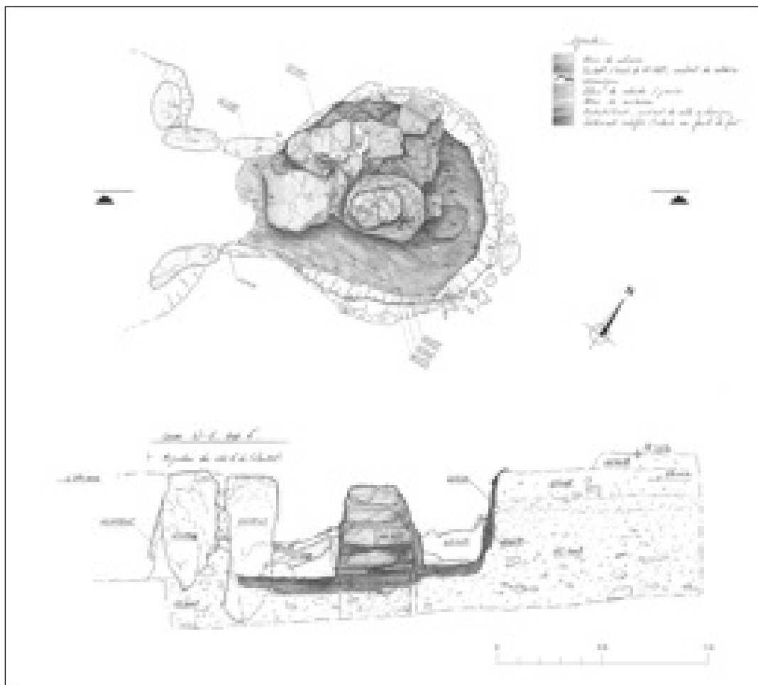
Fig. 2. Vufflens-la-Ville (VD). Relevé en plan et en coupe du four de potier St. 381. Dessin A. Pignolet (Archeodunum SA).
