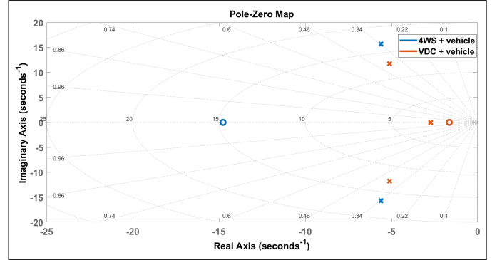
Fig. 6. Poles-zeros analysis.
