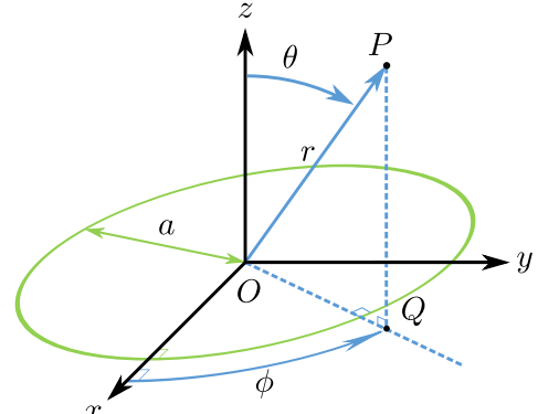
Fig. 2: Current loop parameters
