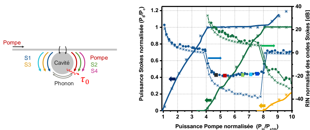
Figure 1. À gauche : Principe de base d'un laser Brillouin multi-Stokes ; à droite : puissance optique des trois premiers ordres de Stokes en fonction de la puissance incidente. Les courbes continues sont les caractéristiques expérimentales ; les points étoiles sont liés à un calcul analytique (caractéristique ou RIN) tandis que les points disques sont des mesures expérimentales de RIN. Les désaccords suivant ont permis de retrouver les valeurs expérimentales : le carré noir correspond à un désaccord \Delta v de 100 kHz, le rouge de 250 kHz, le vert de 400 kHz, le bleu clair de 400 kHz, le bleu profond de 450 kHz.
