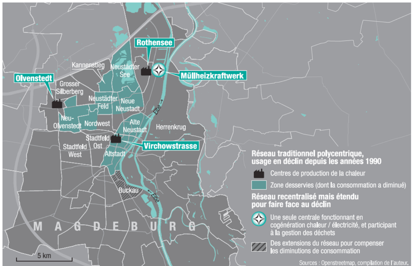
Carte 1. Magdeburg et son système recentralisé du chauffage urbain
