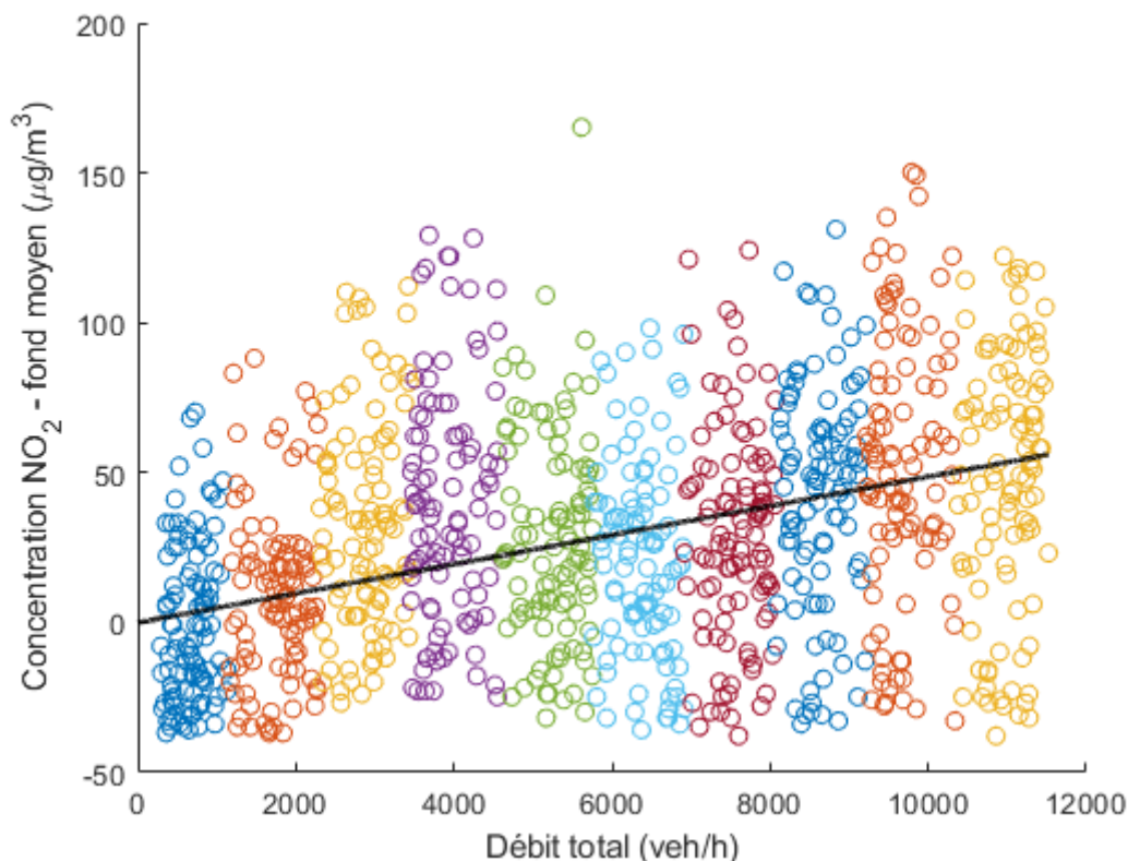
Figure 5 : sélection de 100 observations des couples (débit total, concentration \text{NO}_2 mesurée - fond moyen calculé) pour chacune des 10 classes de débits. La droite correspond à un ajustement linéaire avec valeur nulle à l'origine et une pente de 0.004863 \mu\text{g.h/veh.m}^3 .
