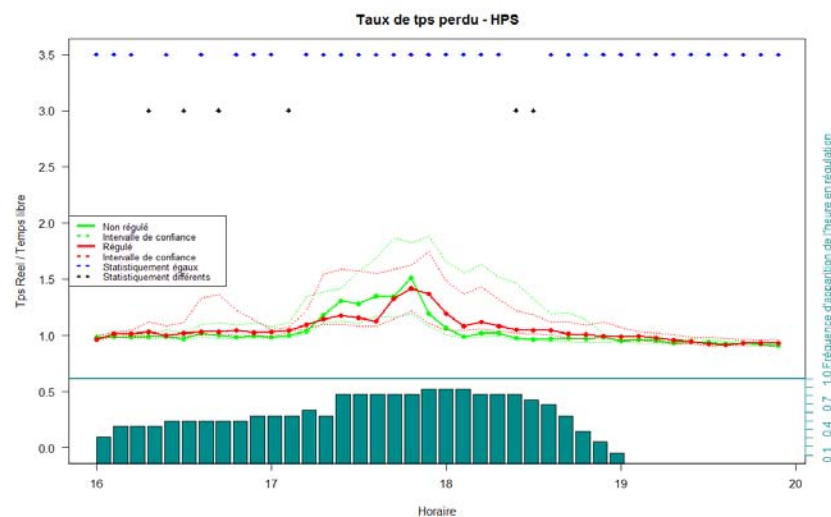
Figure 9 : évolution, en période de pointe du soir, des temps de parcours moyens des périodes régulées et non régulées sur l'ensemble du temps. (Source : auteurs)
