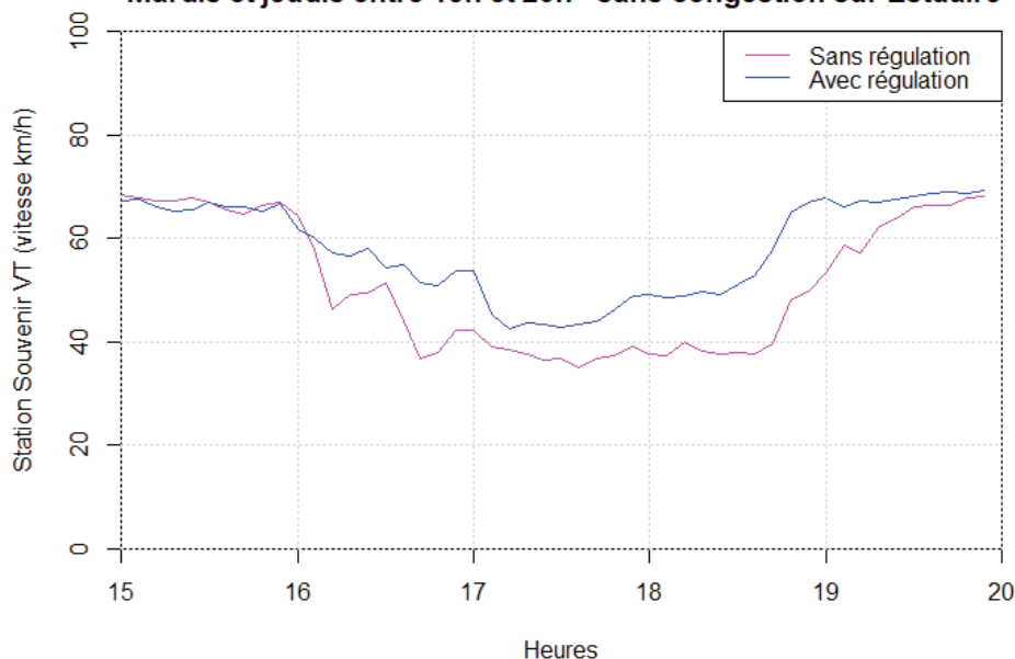
Vitesses moyennes en aval de la porte de Saint-Herblain avec VAE Mardis et jeudis entre 15h et 20h - sans congestion sur Estuaire
