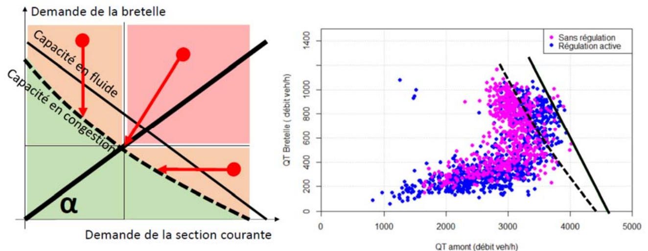
Figure 1 : principes et illustration du fonctionnement d'un convergent. On distingue deux régimes. Le premier est le régime fluide pour lequel la demande totale est inférieure à la capacité. Sur le schéma de gauche, ceci est matérialisé par ligne droite continue correspondant à la « capacité en fluide ». Le second régime est congestionné. Lorsque la congestion est installée, la capacité est réduite (« capacité en congestion »). La figure de droite est obtenue à partir de mesures en aval du convergent de Saint Herblain, sur le périphérique nantais. Chaque point correspond à un débit mesuré pendant une période de 6 minutes, l'abscisse correspond au débit sur le périphérique, l'ordonnée au débit mesuré sur la bretelle.
