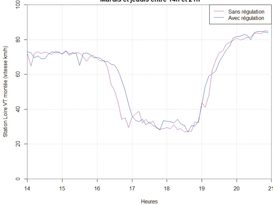
Vitesses moyennes en amont du pincement sur le pont sans VAF Mardis et jeudis entre 14h et 21h
