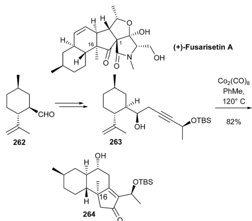
Scheme 60 Li and Yang total synthesis of (+)-fusarisetin A.
