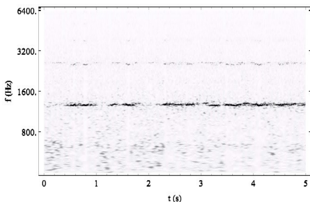
Figure 3: Analyse en ondelettes pendant la phase de sifflement enregistrée sur le microphone N°4.
