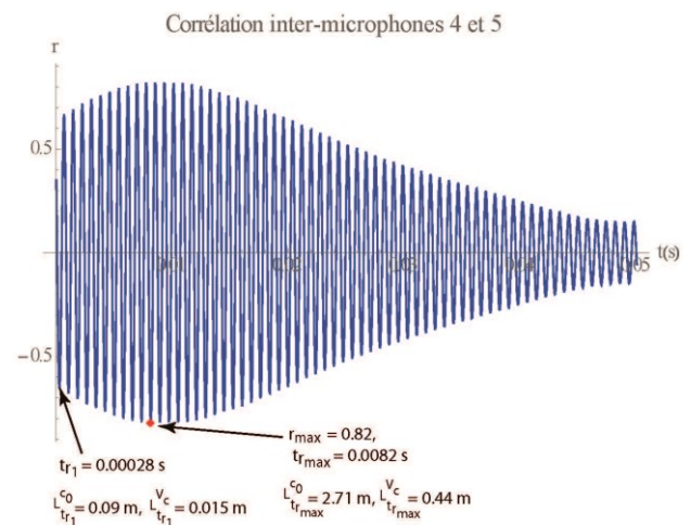
Figure 7 : Corrélation de Pearson entre les micros 4 et 5 calculée entre les instants t = 400 s et t = 450 s (le riser siffle très fortement) pour le signal filtré autour du premier mode transverse du riser par filtre passe-bande entre 800 Hz et 1600 Hz.
