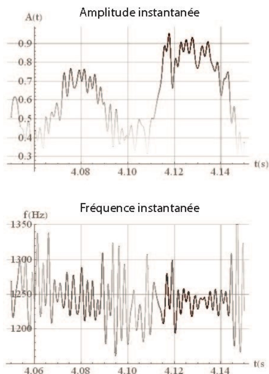
Figure 4 : Amplitude et fréquence instantanées pendant la phase de sifflement enregistrées sur le microphone N°4 pour le signal filtré autour du premier mode transverse du tuyau (filtre passe-bande entre 800 Hz et 1600 Hz).
