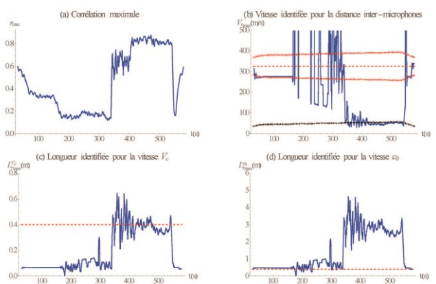
Figure 9 : Analyse de corrélation entre les micros 4 et 5. (a) corrélation au maximum absolu ; (b) vitesse identifiée par la distance inter-microphones divisée par le temps identifié au maximum absolu. (c) longueur identifiée par la vitesse de convection multipliée le temps le temps identifié au maximum absolu. (d) longueur identifiée par la vitesse des ondes multipliée le temps le temps identifié au maximum absolu.
