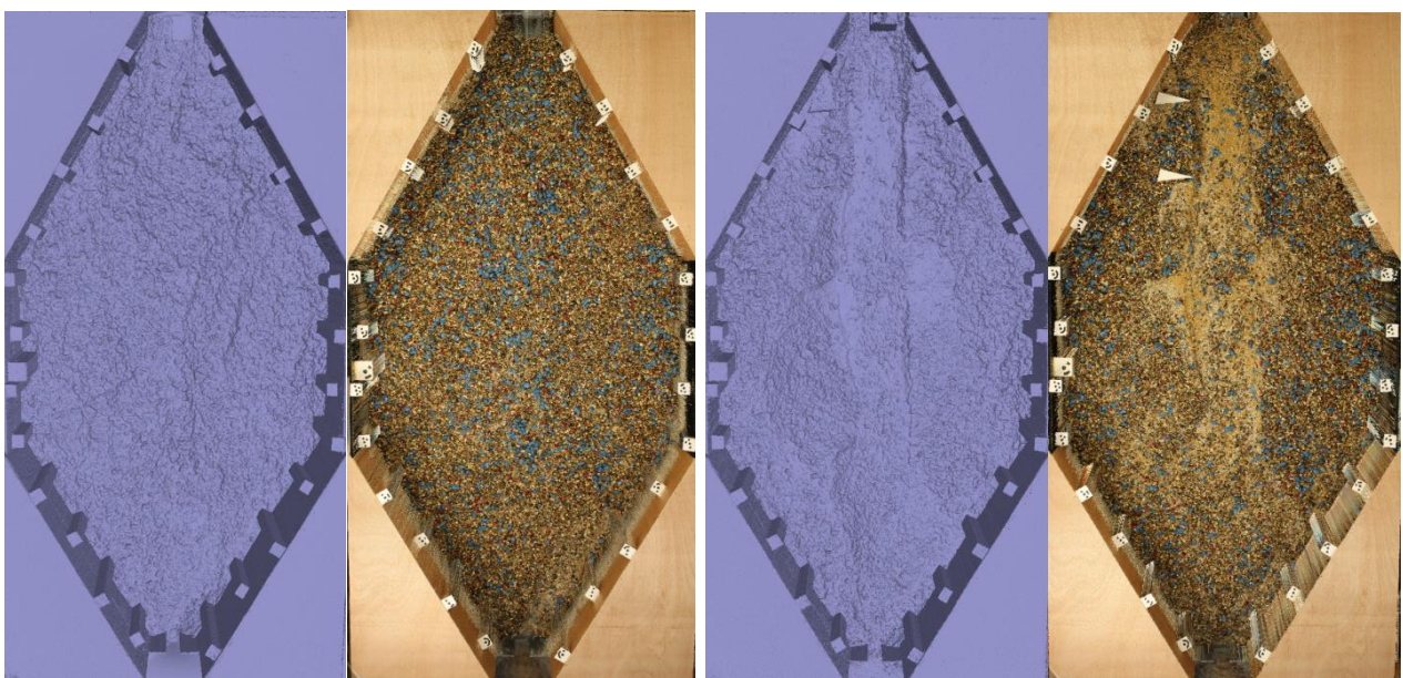
Figure 20 : Détail des morphologies et du tri granulométrique dans deux étapes clés à gauche un faciès d'écoulement en nappe et pavé ; à droite un chenal marqué après une rupture, apparition de la granulométrie fine sous-jacente.
