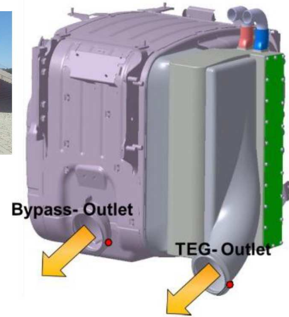
ATS-TEG
