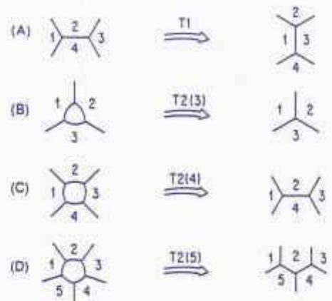
Figure 3 : Les trois processus T_2 décrivent les réarrangements locaux possibles, consécutivement à la disparition d'une bulle à 3, 4, ou 5 côtés. Le processus T_1 , lui, correspond à l'échange de côtés entre quatre bulles et permet de relaxer certaines contraintes mécaniques du système.
