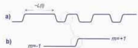
Figure 8 : (a) Coupe schématique d'une configuration de l'aimantation, à un temps donné, pendant l'évolution du modèle d'Ising continu. Les distances entre interfaces sont de l'ordre de L(t) \sim t^{1/2} , alors que leur largeur reste finie. Si on pose m(x,t) = \sigma(l(x,t)) , où le profil à l'équilibre \sigma est défini dans le texte et plus loin, l(x,t) s'interprète alors comme la distance algébrique à l'interface la plus proche. Au même instant, la configuration (plus régulière) de l(x,t) , associée à celle de m(x,t) , est représentée en pointillés. La distribution de probabilité pour l est certainement plus proche d'une gaussienne que celle de m . (b) La forme d'une interface de (a) est localement identique à celle qui séparerait deux domaines infinis purs, à l'équilibre. On montre facilement que ce profil \sigma(l) est donné par d^2\sigma/dl^2 = V(\sigma(l)) , où V est le potentiel défini en équation (4).
