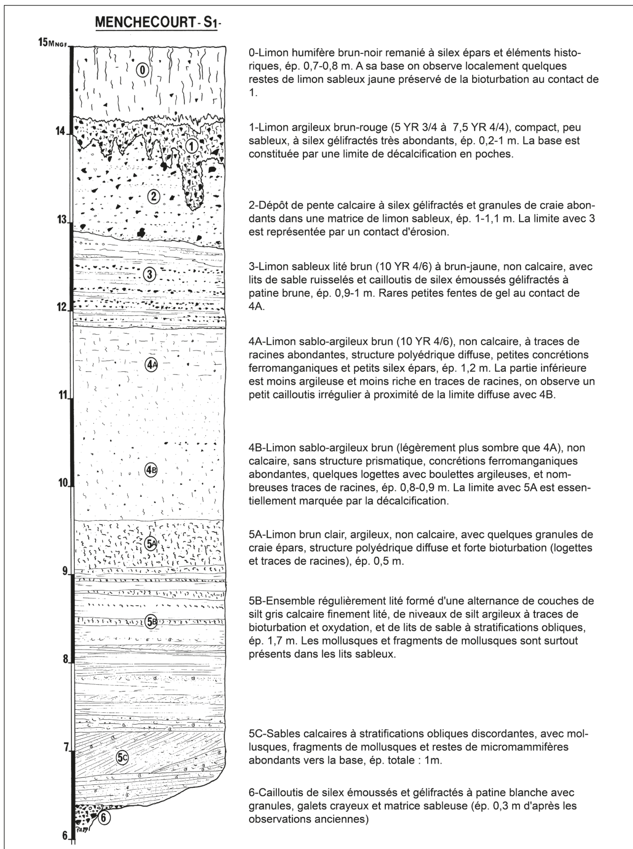
Fig. 10 : Description du sondage S1 réalisé en 1989 à Menhecourt (Antoine, 1990).
