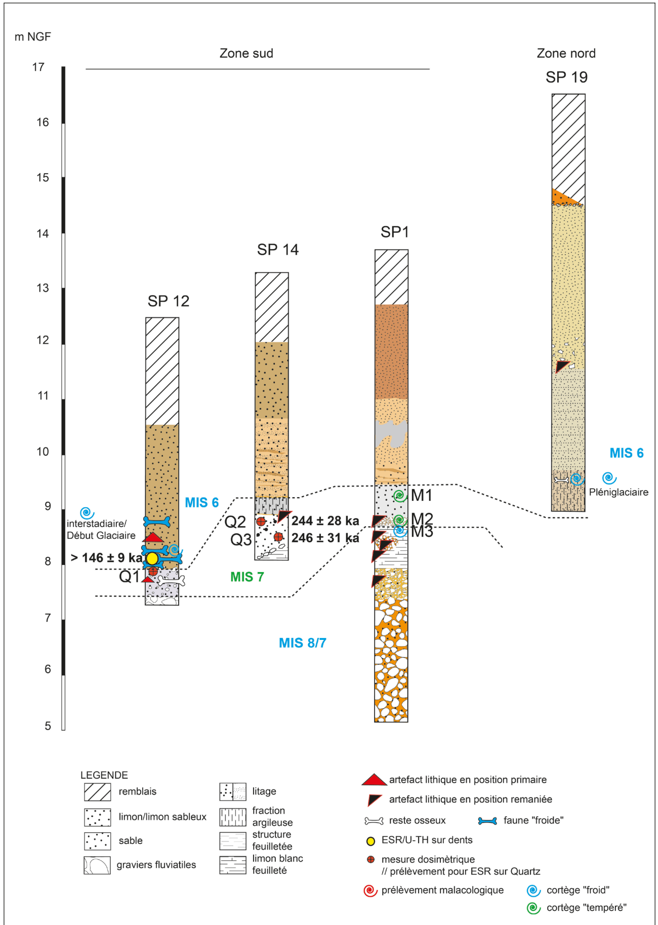
Fig. 9 : Synthèse stratigraphique des données recueillies suite au diagnostic archéologique réalisé sur le site de Menchecourt à Abbeville en 2014.
