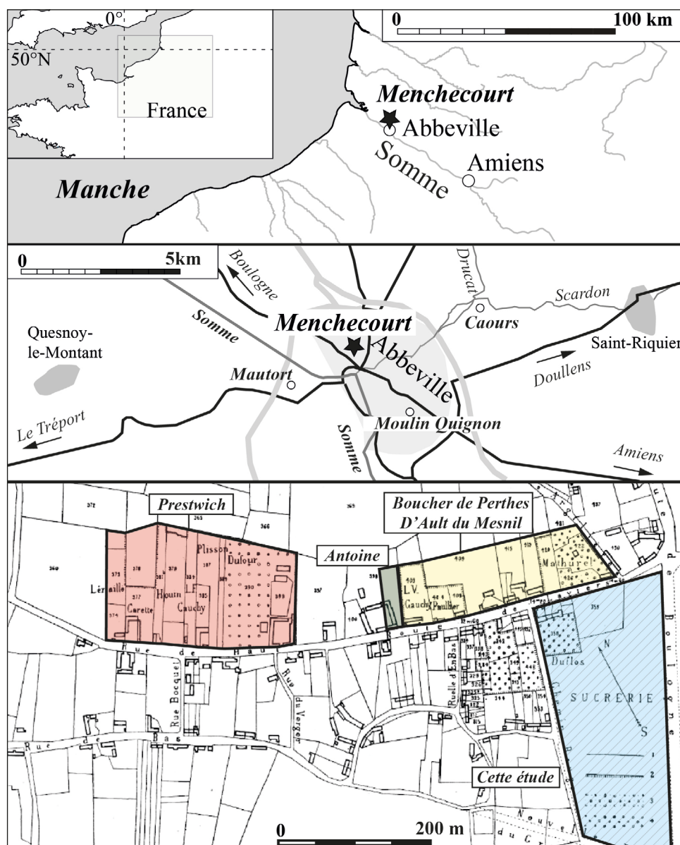
Fig. 1 : Situation géographique du site de Menchecourt (Somme).
