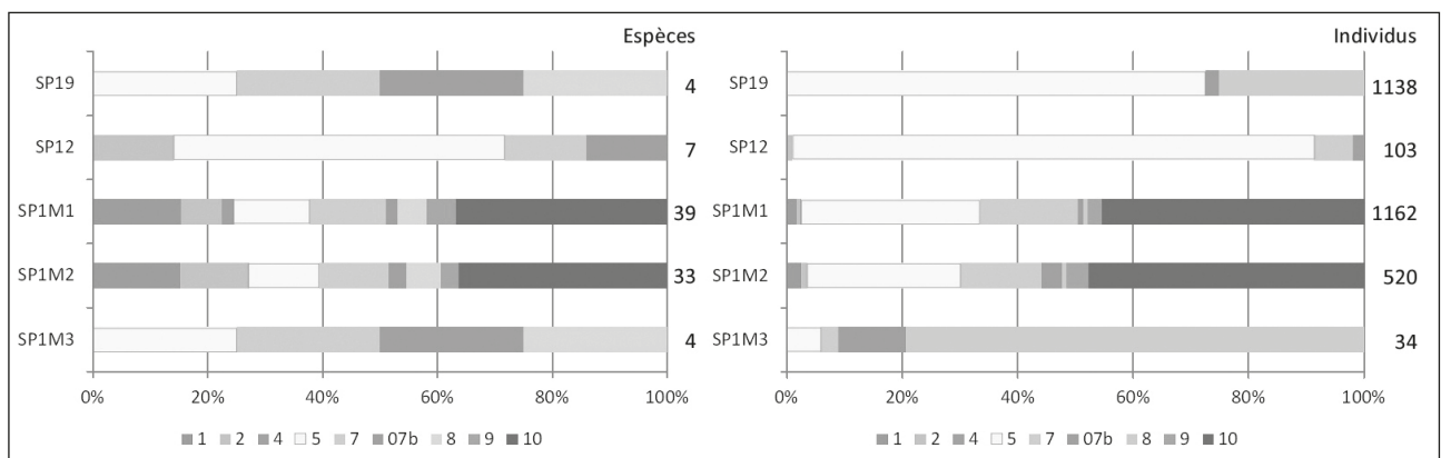
Fig. 8 : Spectres malacologiques de Menhecourt. Groupes écologiques d'après Puisségur (1976).
