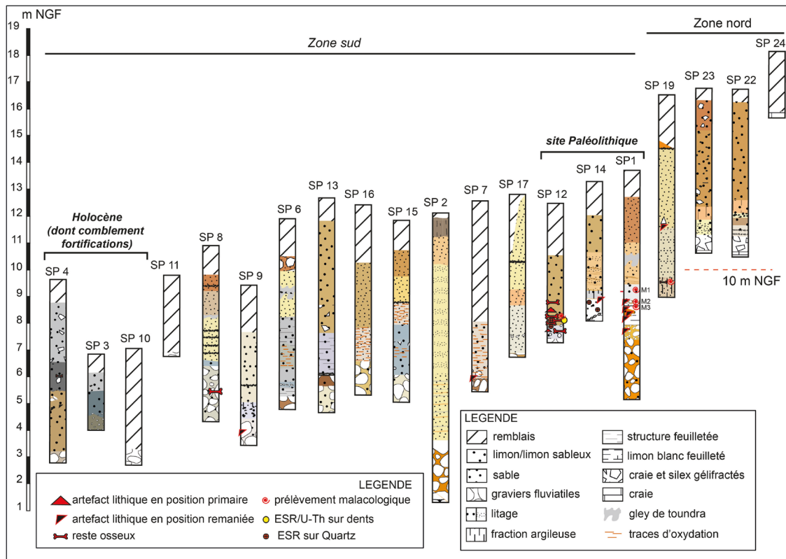
Fig. 5 : Localisation des sondages réalisés à Menhecourt lors du diagnostic archéologique de 2014 et séquences stratigraphiques observées (d'après Loch et Coutard, 2016).
