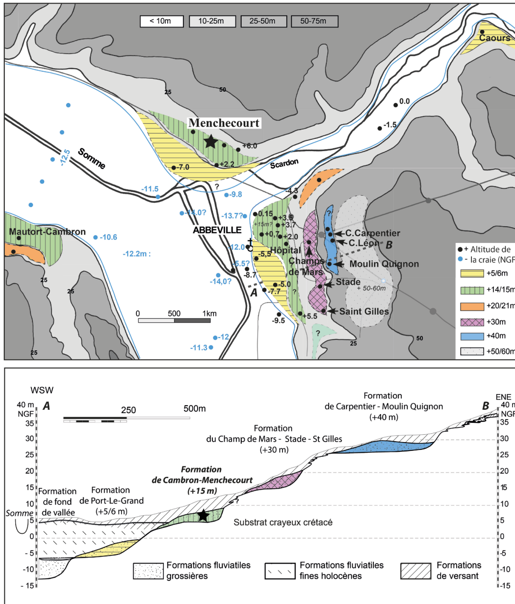
Fig. 4 : Carte et profils des formations alluviales fossiles de la Somme à Abbeville (d'après Antoine et al., 2016, modifié).
